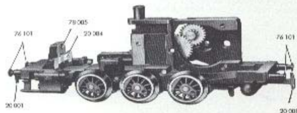
Fig. 3 Treibgestell
