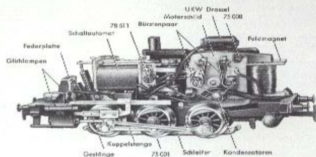
Fig. 2 Fahrgestell
