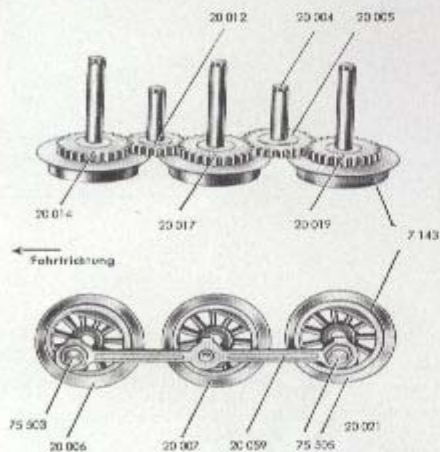
Fig. 6 Gestänge
