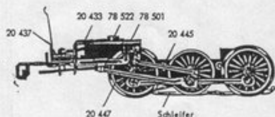
Fig. 2b Bodenstück mit Gestänge
