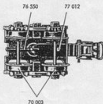
Fig. 4 Drehgestell mit Kupplung (von unten gesehen)
