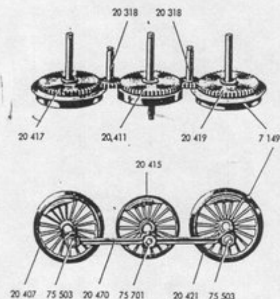
Fig. 6 Drehgestell
