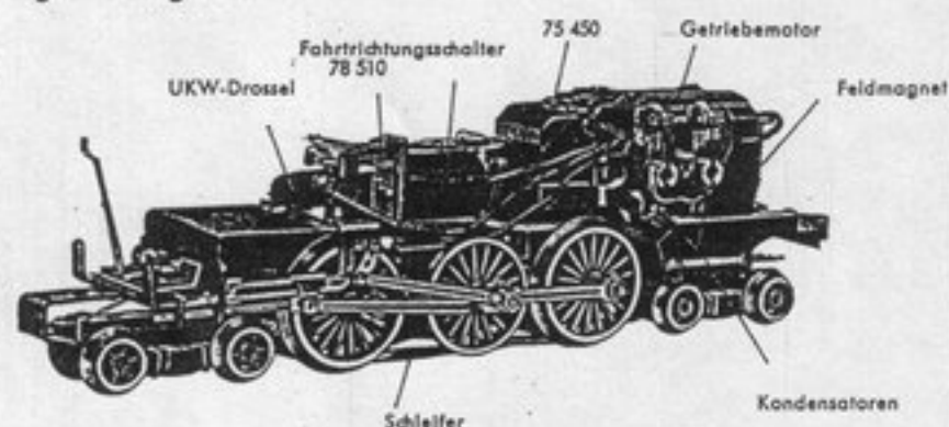
Fig. 2 Fahrgestell
