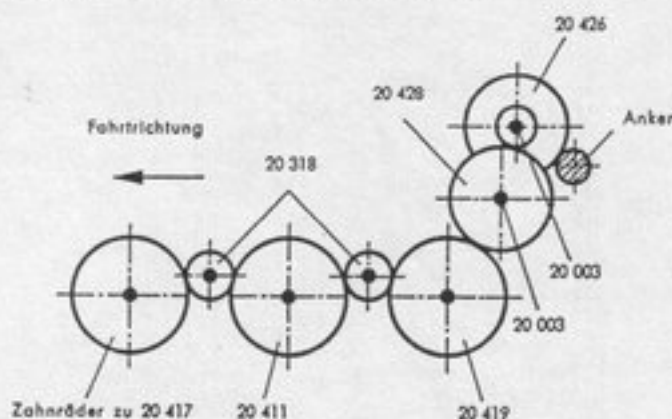
Fig. 5 Treibachsteile und Treibräder
