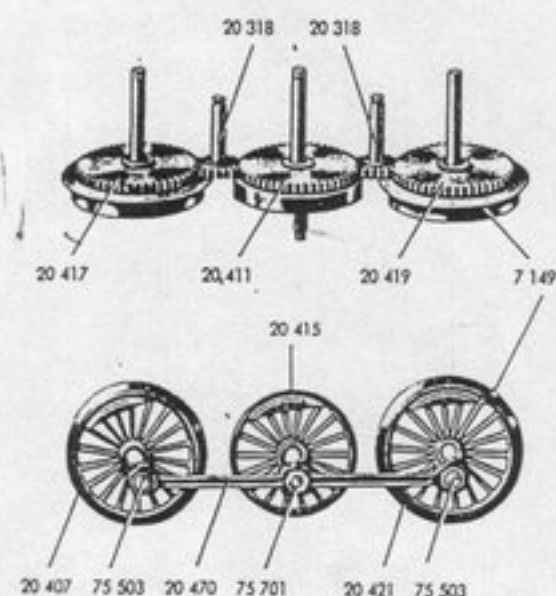
Fig. 6 Drehgestell
