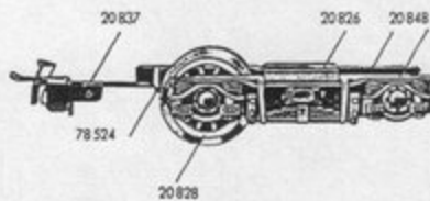
Fig. 6 Laufgestell
