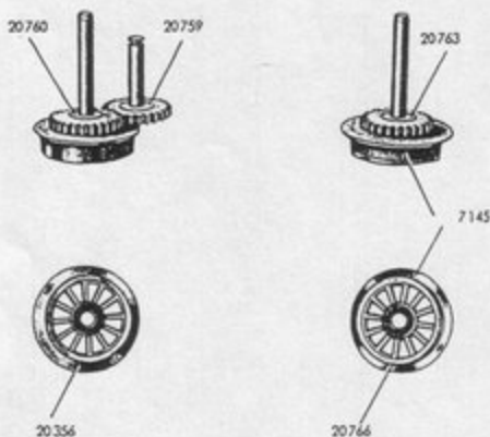
Fig. 6 Laufgestell
