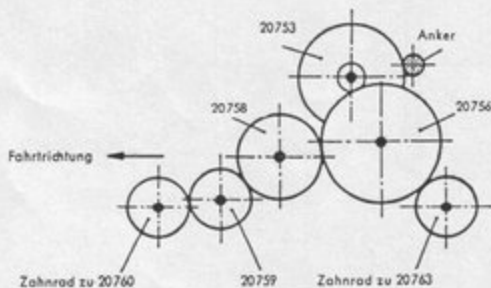
Fig. 5 Treibachse und Treibräder
