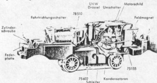
Fig. 3 Treibgestell
