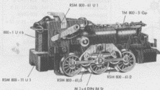
Fig. 6 Fahrgestell RSM 800 (Getriebe Seite)
