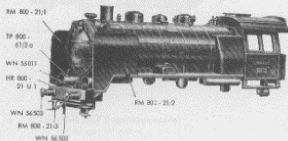
Fig. 2 Lokomotiv-Aufbau RM 800
