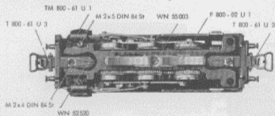
Fig. 3a Lokomotive TM 800 von unten gesehen
