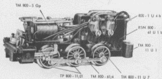
Fig. 3 Fahrgestell TM 800 und RM 800
