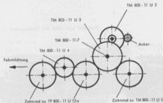
Fig. 8 Anordnung der Getrieberäder bei den drei Lokomotiven gleich
